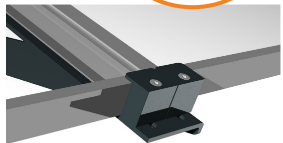
Cavalier de verrouillage panneaux par l'extérieur Fabrication sur mesure suivant l'épaisseur du panneau
