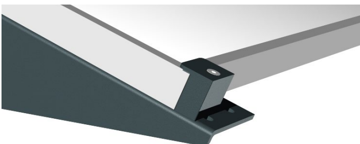
Cavalier de verrouillage panneaux par l'extérieur Fabrication sur mesure suivant l'épaisseur du panneau
