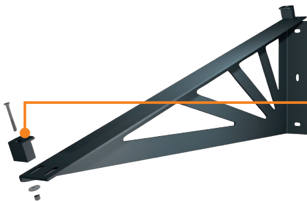
Cavalier de verrouillage panneaux par l'extérieur Fabrication sur mesure suivant l'épaisseur du panneau
